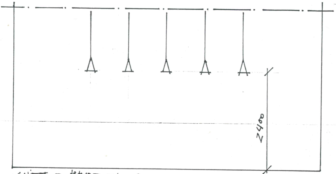
SNITT - HØYDE TAVLES
