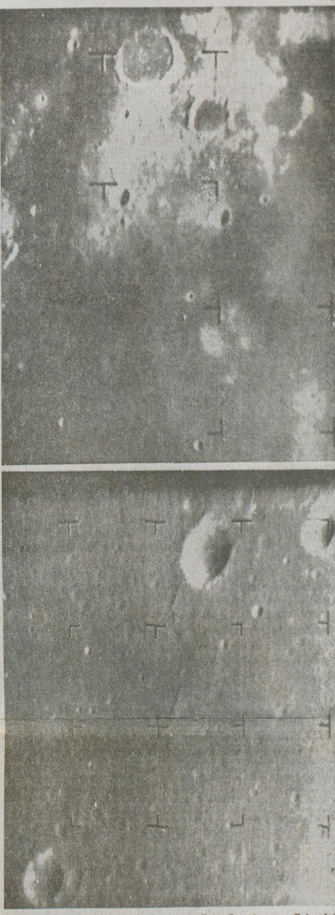
To av bildene som ble tatt av månens overflate. Øverst er overflaten fotografert i en avstand av 750 km, og bildet dekker et område på 120 kvadratkilometer. De minste kratere her er litt over 200 meter i diameter. — Nederst overflaten fotografert i en avstand av 40 km. De minste kratere her er litt over 20 meter i diameter.
